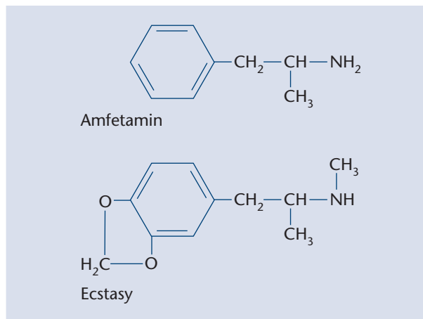
Figur 32. De kemiske formler for ecstasy og amfetamin. Fysiologibogen – den levende krop Tegning: Erik Hjørne © Nucleus Forlag 2006
