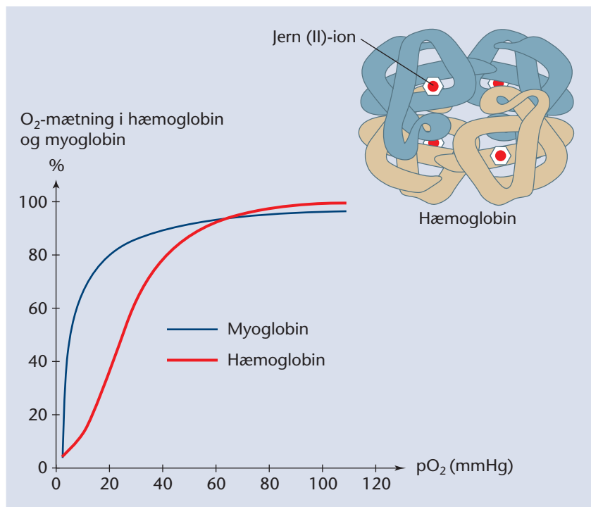
Figur 50. Iltbindingskurver for hæmoglobin og myoglobin. Fysiologibogen – den levende krop Tegning: Erik Hjørne © Nucleus Forlag 2006
