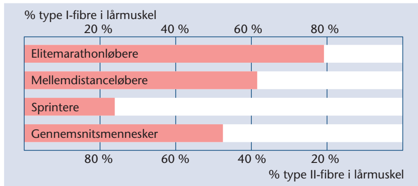
Figur 96. Procentvis fordeling af fibertyper. Fysiologibogen – den levende krop Tegning: Erik Hjørne © Nucleus Forlag 2006
