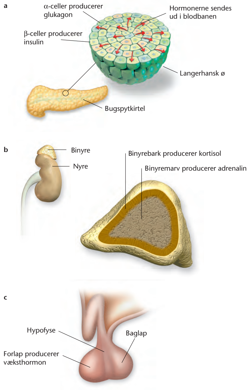
Figur 180. a. Bugspytkirtel med \alpha - og \beta -celler. b. Binyre med marv og bark. c. Hypofyse. Fysiologibogen – den levende krop Tegning: Henning Dalhoff © Nucleus Forlag 2006
