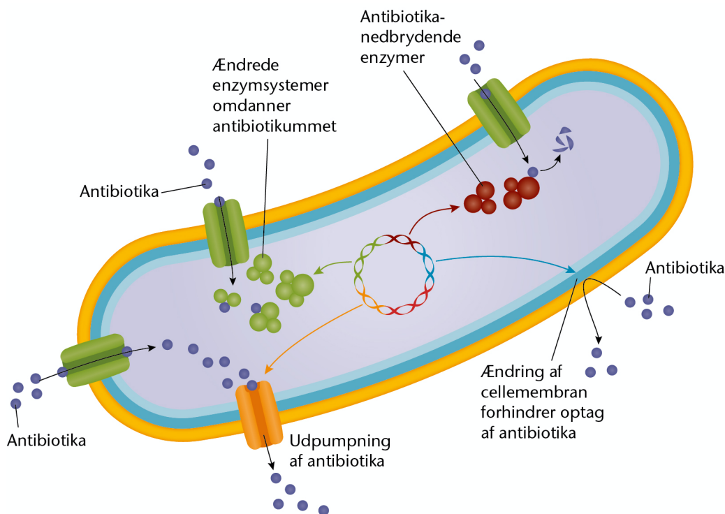
Figur 1. Resistensmekanismer.
