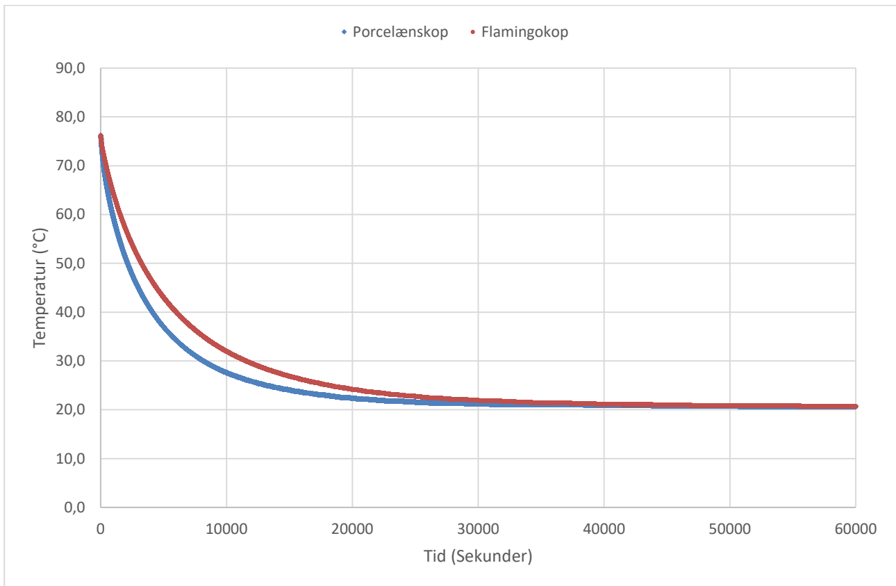
Figur 1. Temperaturens ændring over tid i vandet i kopper af forskelligt materiale.
