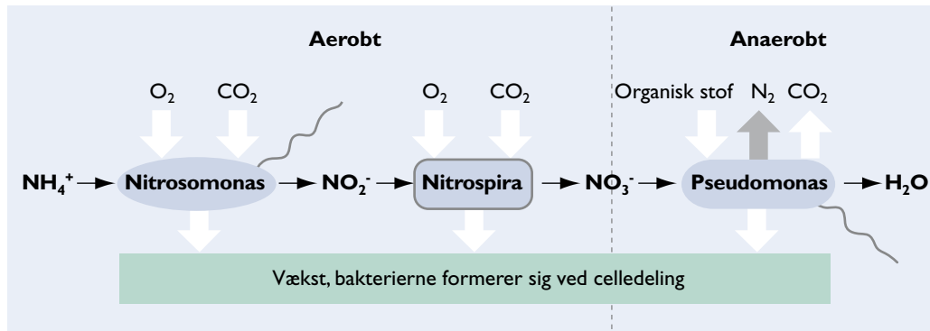
Figur 36. Udsnit af N-kredsløbet. Figuren er rettet i bogens 2. udgave, 2. oplag: \text{CO}_2 -pilen ved Pseudomonas er vendt så den peger ud. Tegning: Erik Hjørne.
